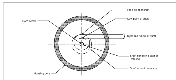
Fig. 4 : Shaft runout
