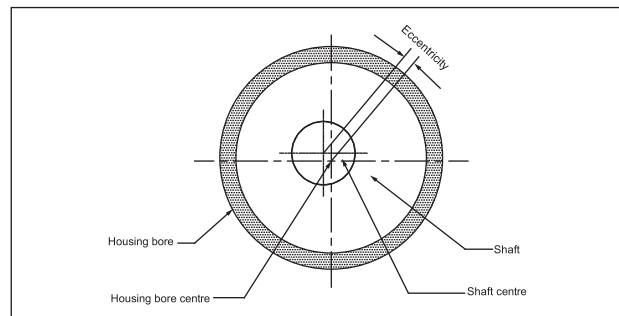
Fig. 3 : Shaft eccentricity
