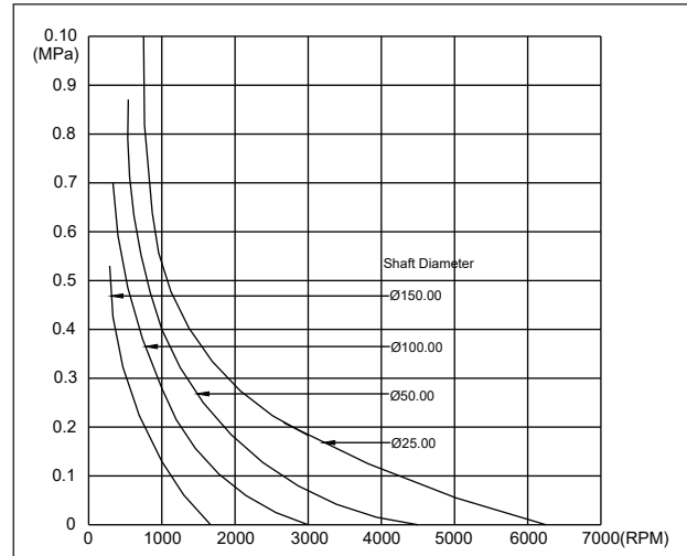
Fig. 8 : Permissible overpressure.
